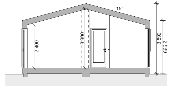
1:100 Snitt A
