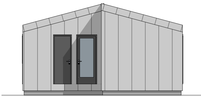
1:100 Fasade Øst
